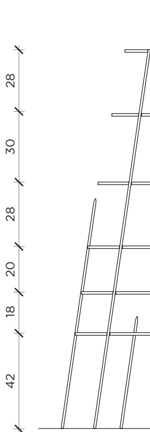
LATO | SIDE
